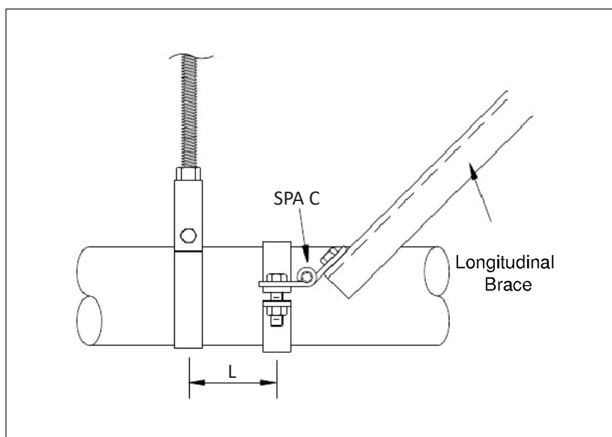
Longitudinal Brace
